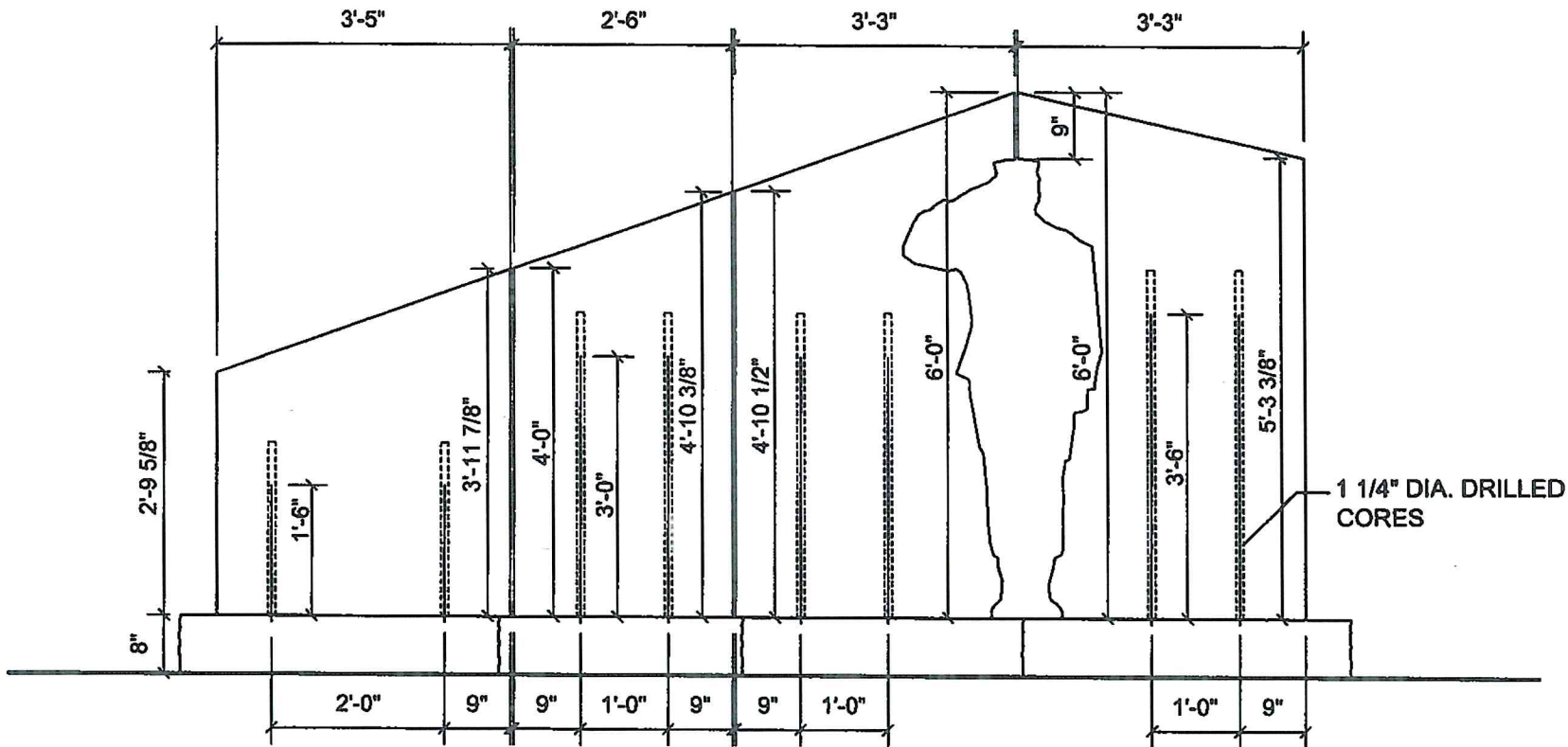
ELEVATION 2
